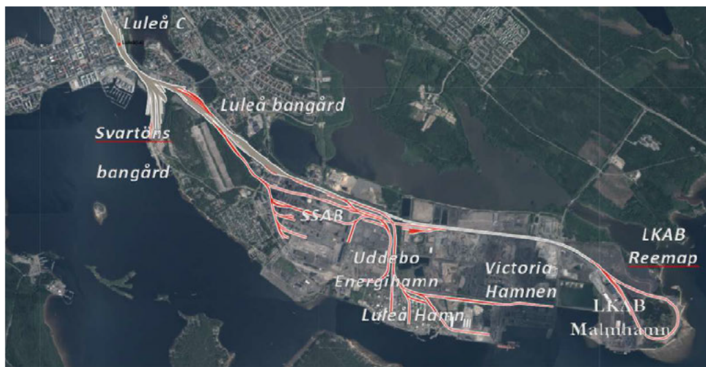
Översiktsbild av dagens järnvägssystem på Svartön. (Bild från NJDB, Trafikverket.)
